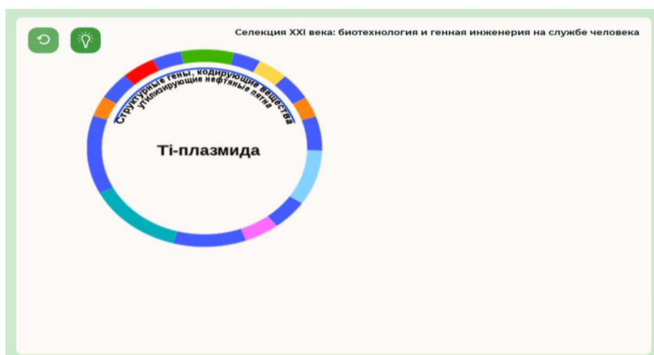
Т-плазида с новыми структурными генами
